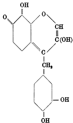
Hämatein
